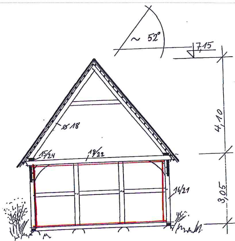
SCHNITT
